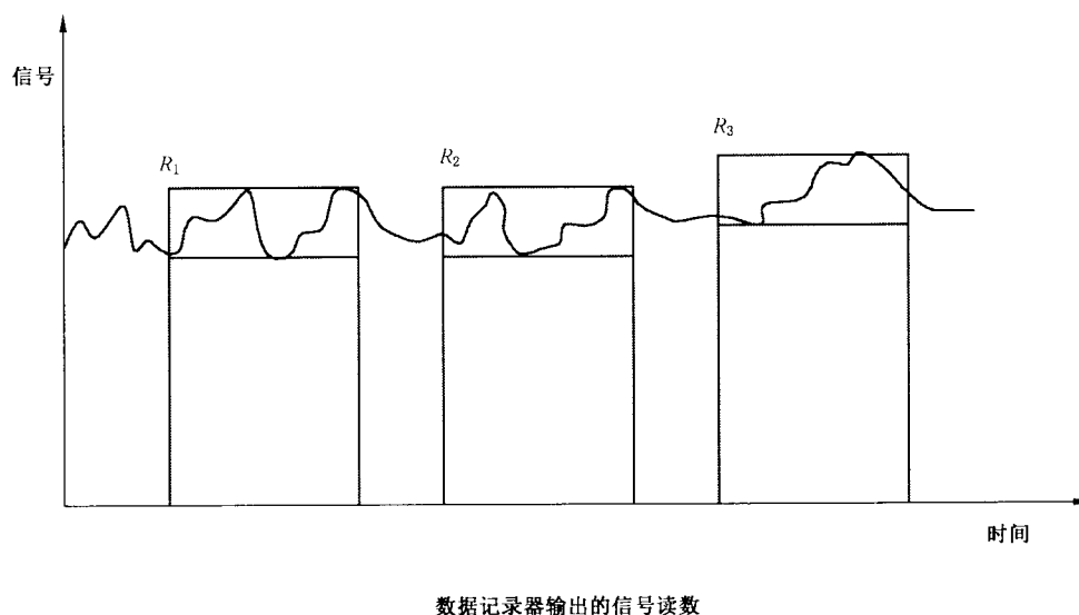
图 B.3 数据记录器输出的信号读数
