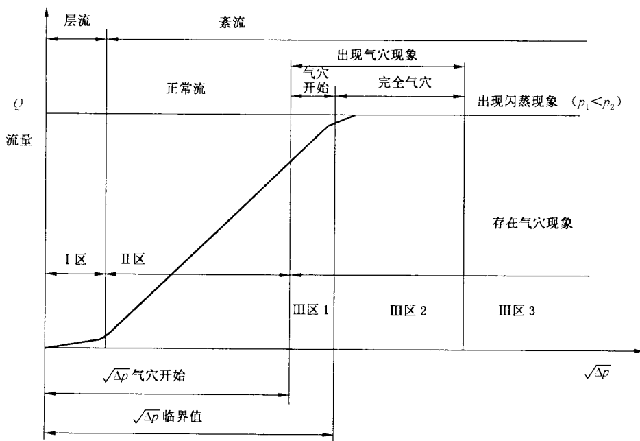
图 A.1 流量相对压力降平方根的曲线图
